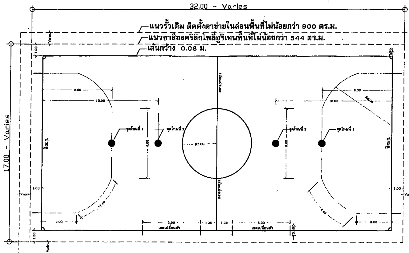
ผังบริเวณปรับปรุงฟุตซอล โรงเรียนเทศบาลคันทรง scale 1 : 150
