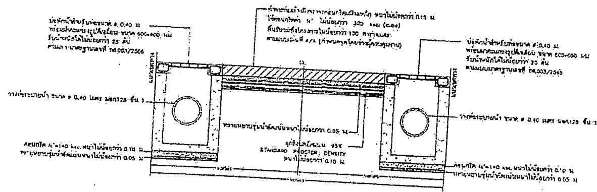
รูปตัด 2 (ใหม่) NOT TO SCALE
