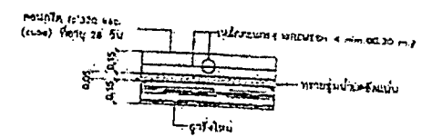
ขยายไหล่ทาง คสล.หนาไม่น้อยกว่า 0.15 ม. NOT TO SCALE
