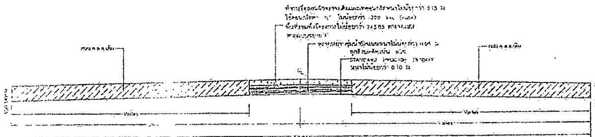
รูปตัด 2 ขนาด 1:20
