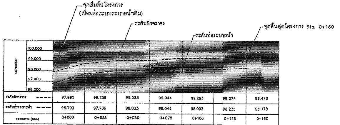
ตารางแสดงค่าระดับและระยะทาง (ซอยกินนุส 2) จาก sta. 0+000 ถึง sta. 0+160
