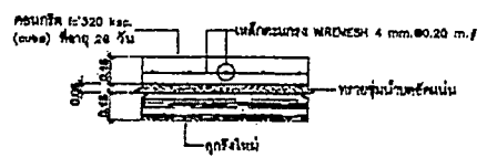
ขยายดินผิวหลังท่อ ค.ส.ล. หน้าไม้ไม่น้อยกว่า 0.15 ม. NOT TO SCALE
