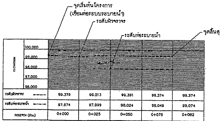
ตารางแสดงค่าระดับและระยะทาง (ซอยกินนุส 2 แยกขวา ซอย 1 ผังขวา) จาก sta. 0+000 ถึง sta. 0+082
