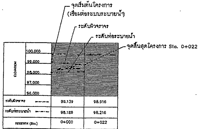
ตารางแสดงค่าระดับและระยะทาง (ซอยเทพารักษ์ 7) จาก sta. 0+000 ถึง sta. 0+022
