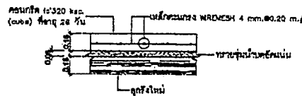
ขยายดินผิวหลังท่อ ค.ส.ล.หนาไม่น้อยกว่า 0.15 ม. NOT TO SCALE
