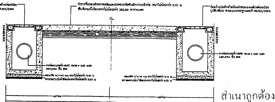
รูปตัด 5 (ใหม่) NOT TO SCALE
