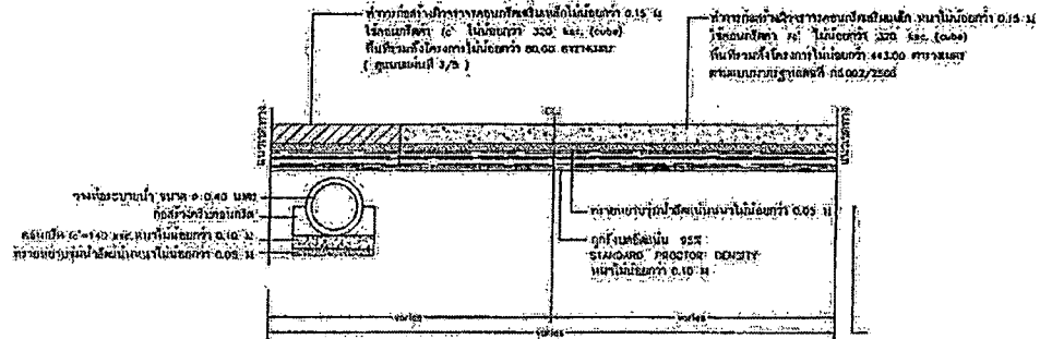
รูปตัด ๑ (ใหม่) NOT TO SCALE
