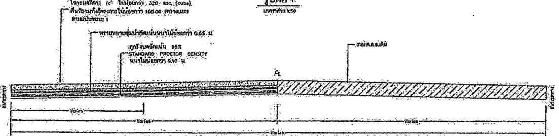
รูปตัด 2 ขนาด 1:50
