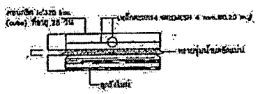
ขยายไหลทาง ค สล หน้าไม่น้อยกว่า 0.15 ม. NOT TO SCALE
