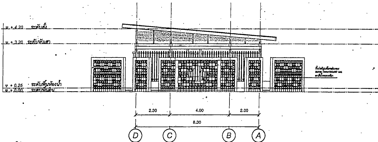
รูปด้าน B มาตรฐาน 1:100
