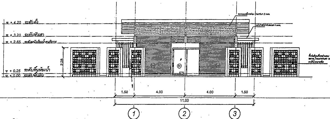
รูปด้าน A มาตรฐาน 1:100
