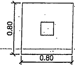
ฐานรากรั้ว, เสาตอม่อ(F2, C2)
