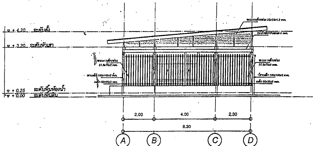
รูปด้าน D มาตราส่วน 1:100
