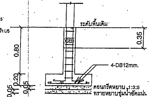
ฐานรากรั้ว, เสาตอม่อ(F2, C2)
