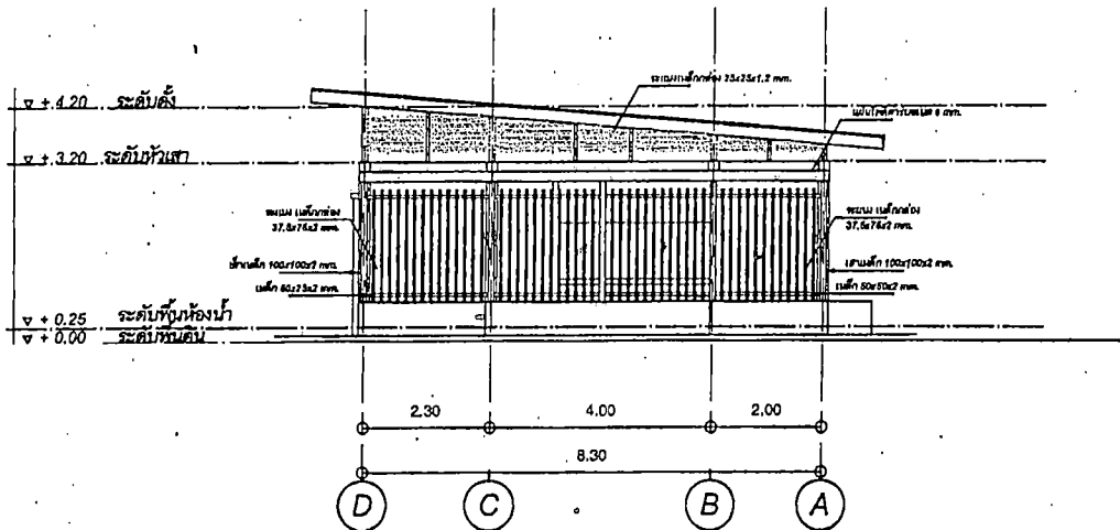
รูปด้าน B มาตราส่วน 1:100
