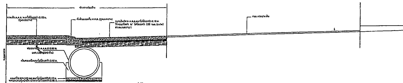
รูปตัด 1 NOT TO SCALE
