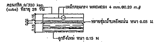
ขยายโหลทาง ค.ส.ล.หนาไม่น้อยกว่า 0.15 ม. NOT TO SCALE
