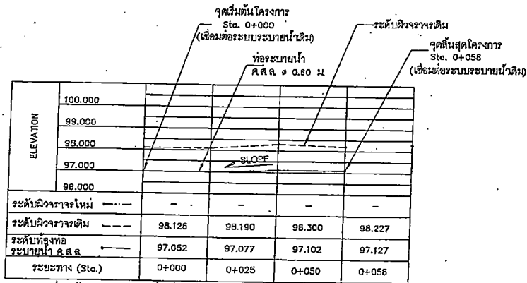
ตารางแสดงค่าระดับและระยะทาง (ช่วงที่ 2) จาก sta. 0+000 ถึง sta. 0+058
