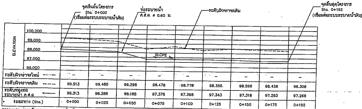
ตารางแสดงค่าระดับและระยะทาง (ช่วงที่ 1) จาก sta. 0+000 ถึง sta. 0+192
