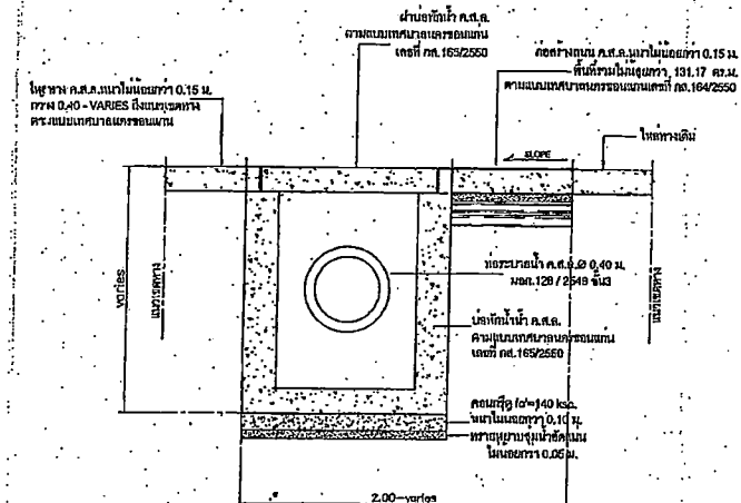
รูปตัด 2 NOT TO SCALE
