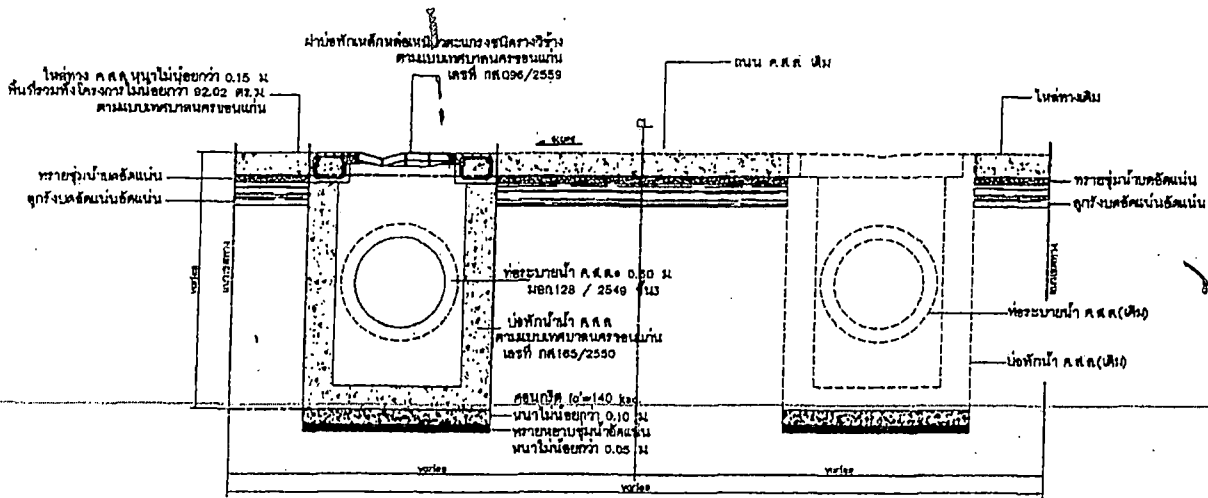
รูปตัด 1 NOT TO SCALE
