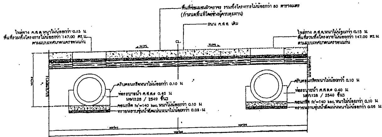
รูปตัด 2 NOT TO SCALE
