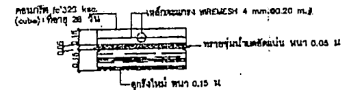
ขยายให้ทาง ค.ส.ต.หนาไม่น้อยกว่า 0.15 ม. NOT TO SCALE
