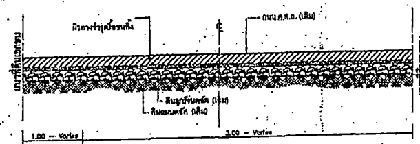
รูปตัด ข-ข (เดิม) มาตราส่วน NTS.
