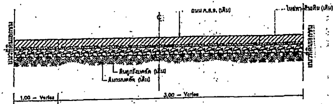
รูปตัด ก-ก (เดิม) มาตราส่วน NTS.
