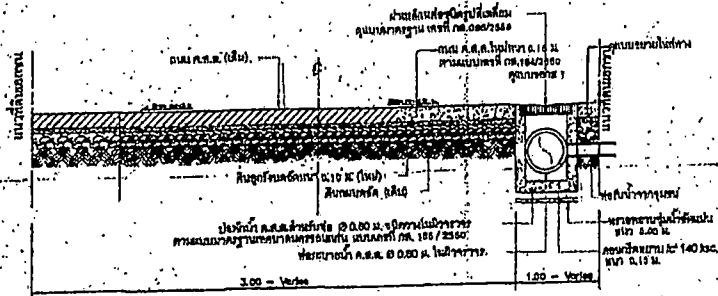
รูปตัด ข-ข (ใหม่) มาตราส่วน NTS.
