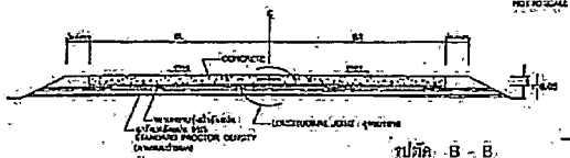
รูปตัด B-B NOT TO SCALE
