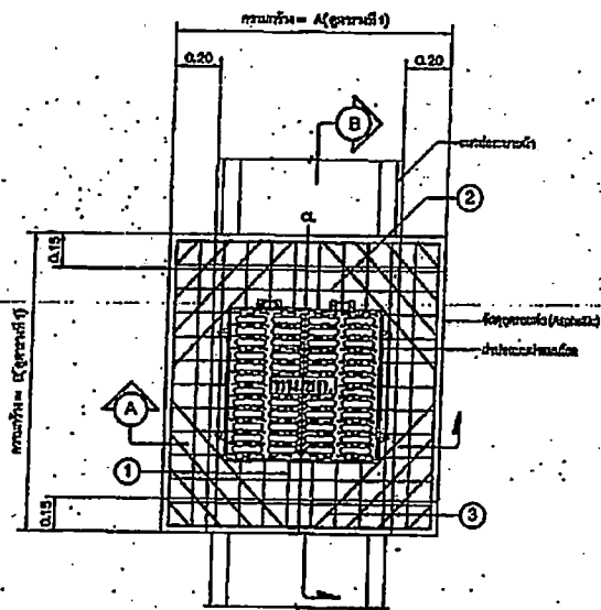
แปลนหลักเสริมโครงสร้างปิดผ่านเหล็กหล่อเทียว NOT TO SCALE
