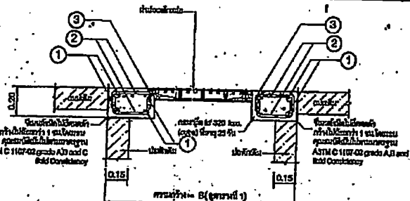
រូបភាព B-B NOT TO SCALE
