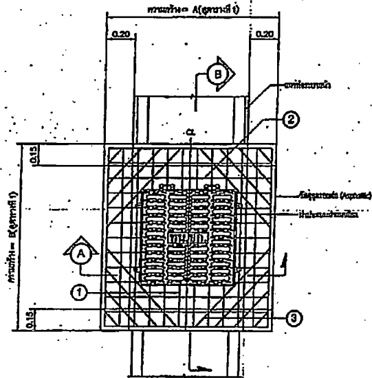
แปลนเหล็กเสริมโครงสร้างปิดฝ่าปอเหล็กหล่อเหนียว
