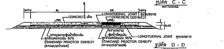
รูปตัด C-C NOT TO SCALE
