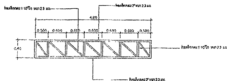
แปลนขยาย TRUSS 1
