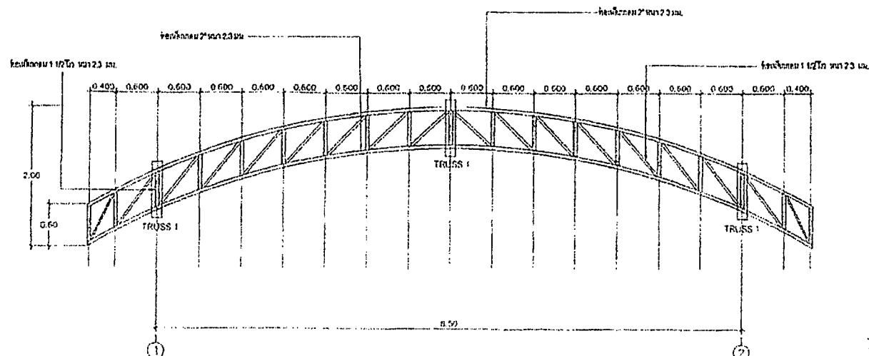
แปลนขยาย TRUSS 2
