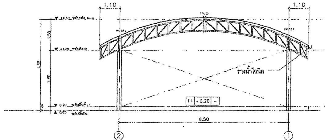
รูปด้าน 3 มาตราส่วน 1 : 75
