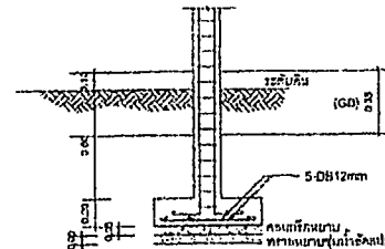
เสาตอม่อ(C1)
