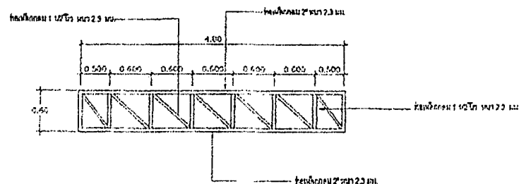
แปลนขยาย TRUSS 1 มาตราส่วน 1 : 50
