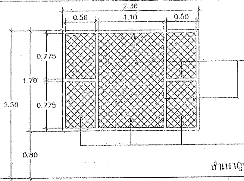
แบบขยายแปลงตามหลัก 2 SCALE 1:25
