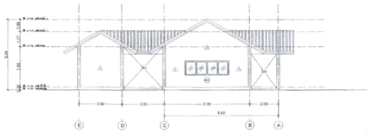
รูปตัด - B
