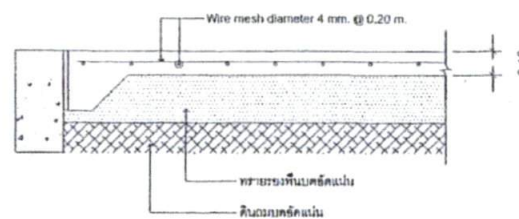
ขยายพื้นวางบนดิน GS
