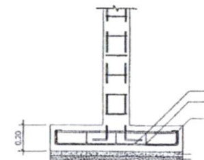
แบบขยาย F1
