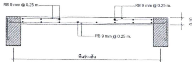
ขยายแผ่นพื้น S1 (พื้นช่วงเดี่ยง)
