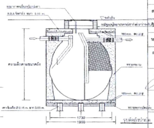
แบบมาตรฐานการติดตั้งถังน้ำบาดาล (ปรับเปลี่ยนได้ตามขนาดและรุ่นของถังน้ำบาดาล)
