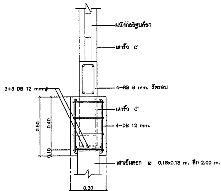
แบบขยายฐานราก F1
