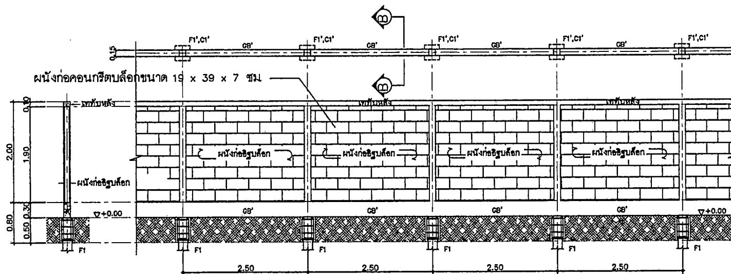
รูปตัด B แบบขยายรั้วแนว B
