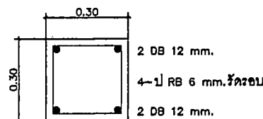
แบบขยายต่อม่อ
