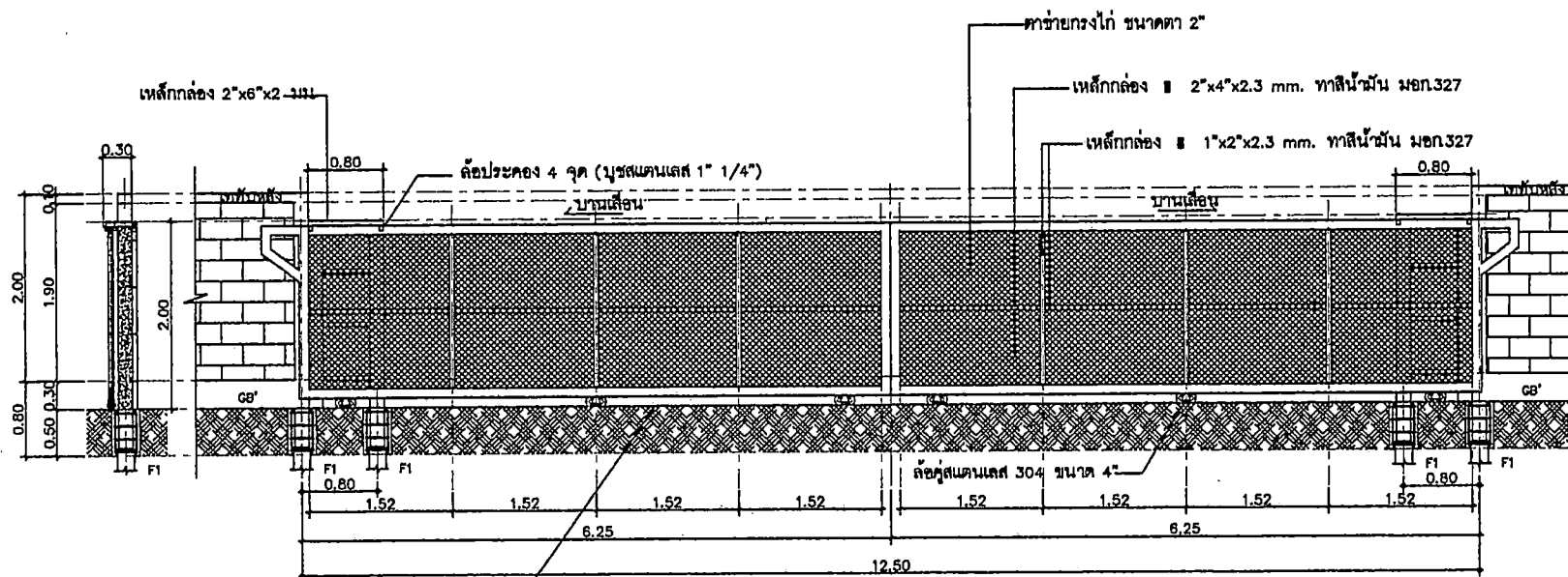
แบบขยายประตู scale : ไม่กำหนด
