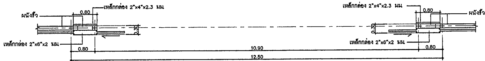
แบบขยายแปลนด้านบน scale : ไม่กำหนด
