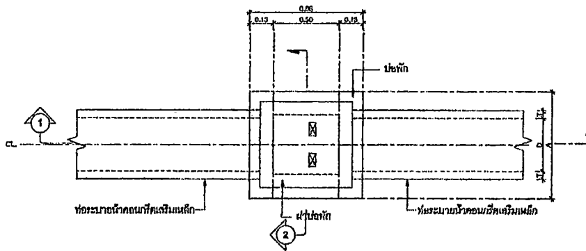
แปลนท่อระบายน้ำในทางเท้า ขนาด Ø 0.30 ม. มาตราส่วน 1:20
