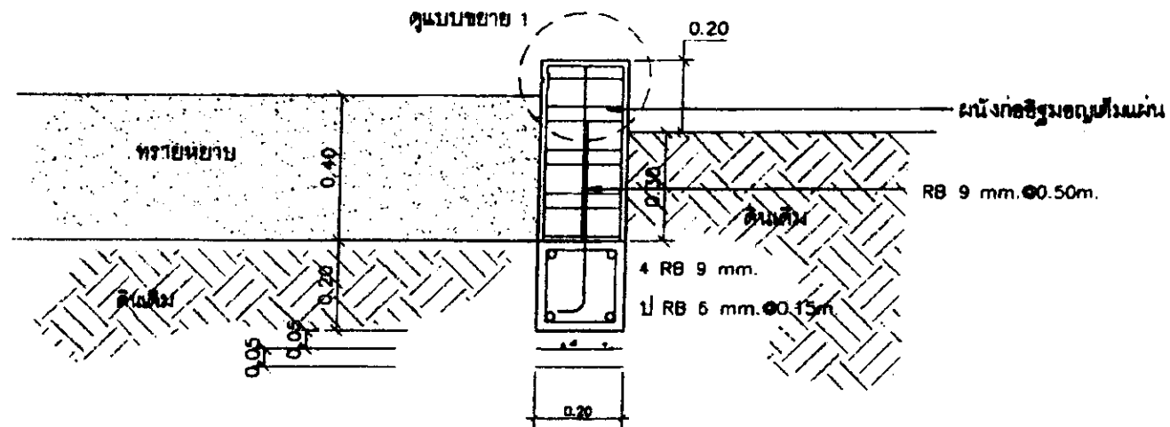
แบบขยายฐานรากแผ่ต่อเนื่องรับกำแพงกันดิน
