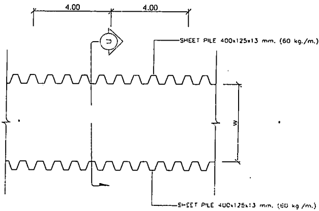
แปลน NOT TO SCALE
