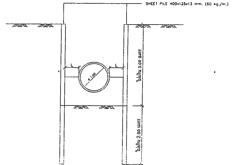
รูปตัด ก NOT TO SCALE
