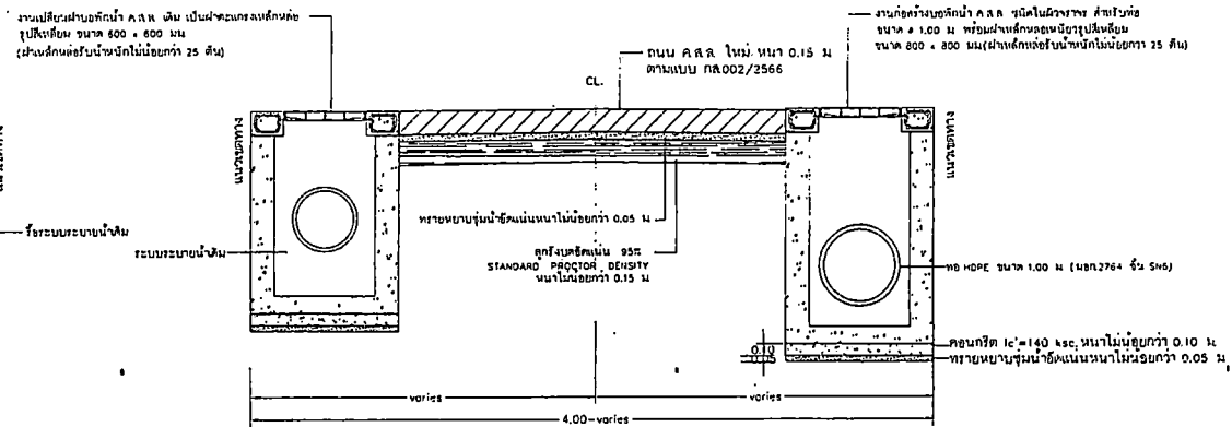
รูปตัด 2 (ใหม่) NOT TO SCALE
