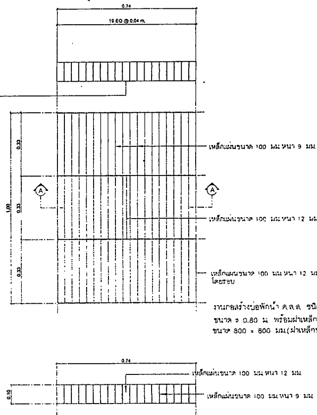
แปลนรางระบายน้ำรูปตัว Y ค.ล.ล. + แปลนขยายเหล็กตะแกรงฝารางยู
