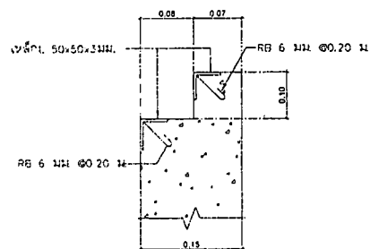
แบบขยาย A Not to scale
