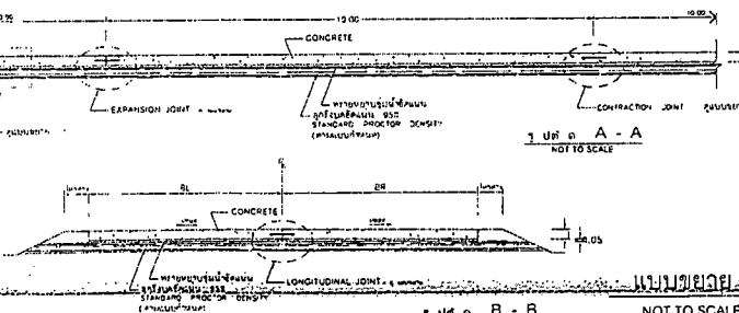
รูปตัด B-B
