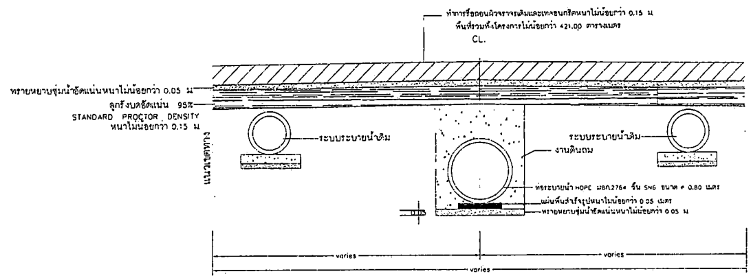
รูปตัด 1 (ใหม่)
