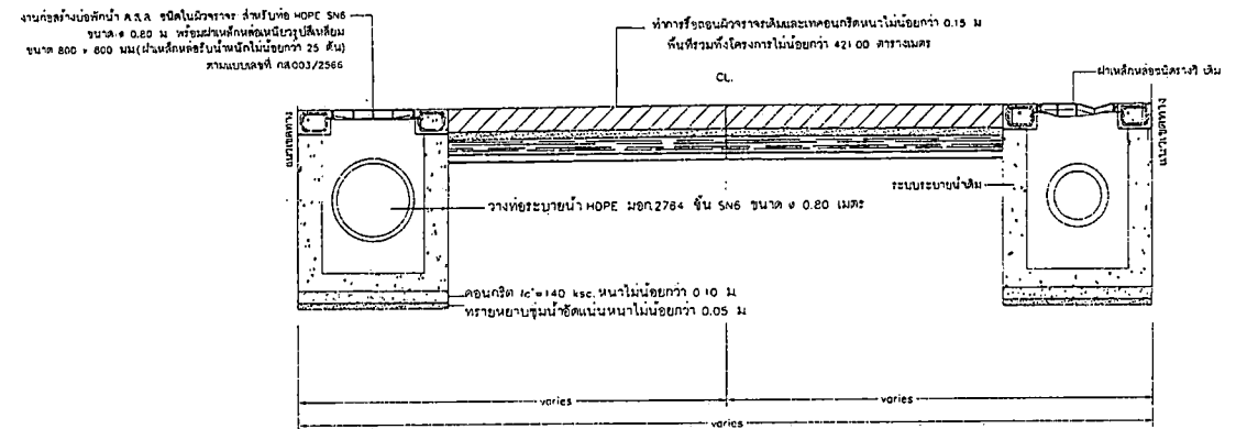
รูปตัด 3 (ใหม่) NOT TO SCALE
