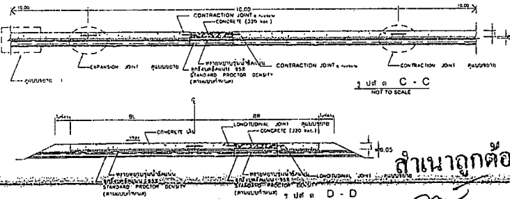
รูปตัด D-D
