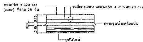
ขยายไหล่ทาง ค.ล.ล. หน้าไม่น้อยกว่า 0.15 ม. NOT TO SCALE
