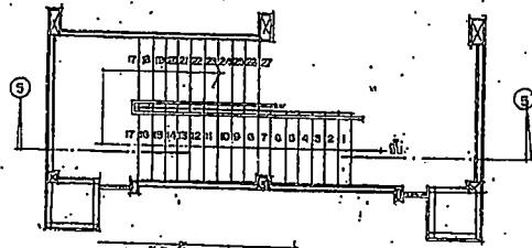
แปลนบันได ชั้นล่าง 1:50
