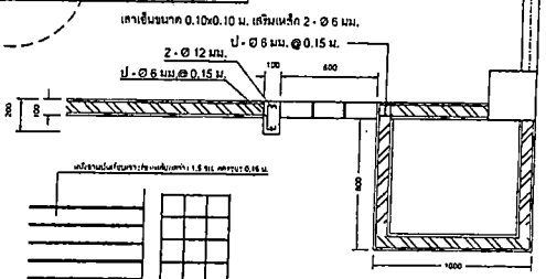
รูปตัดขยาย 2-2
