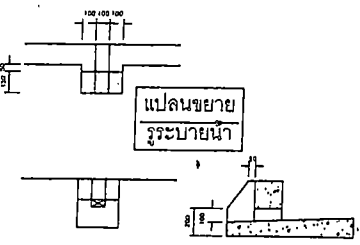
รูปด้าน รูปตัด รูปขยาย A
