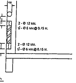
รูปตัดขยาย 2-2
