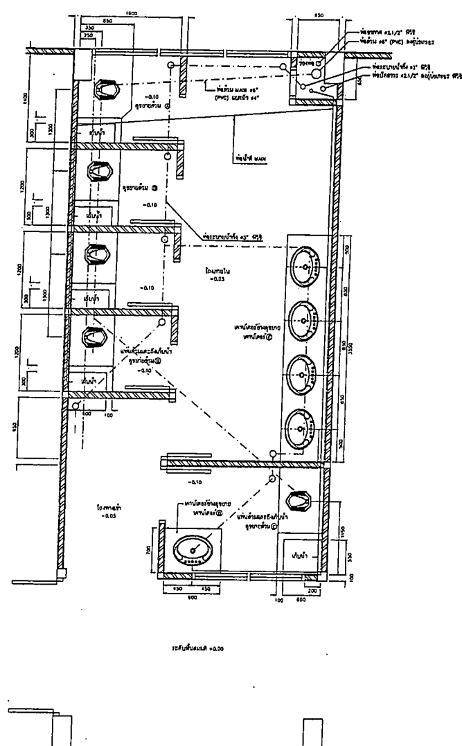
แปลนขยายห้องน้ำหญิงชั้น 2
