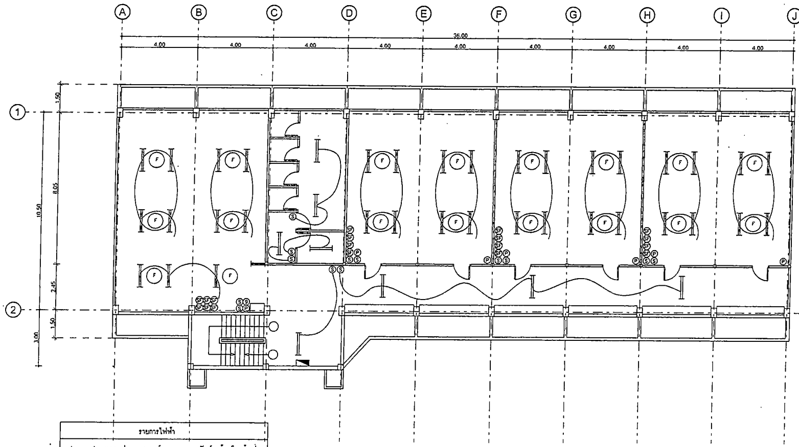
แปลนไฟฟ้าชั้น 2-3-4 1:100
