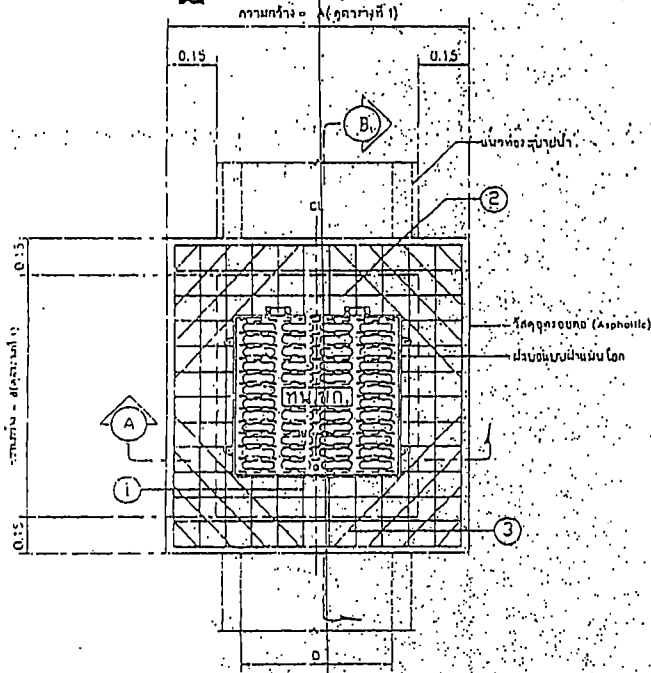
แปลนเหล็กเสริมโครงสร้างยึดผาปอเหล็กหล่อเหนียว
