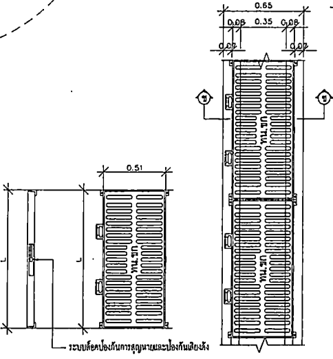
แปลนวางระบายน้ำคู่อัดยว ค.ส.ล. + ฝาดะแกรงเหล็กหล่อระบายน้ำ มาตราส่วน 1/15
