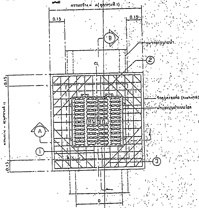
แปลนเหล็กเสริม โครงสร้างยึดพาบ่อเหล็กหล่อเหนียว NOT TO SCALE
