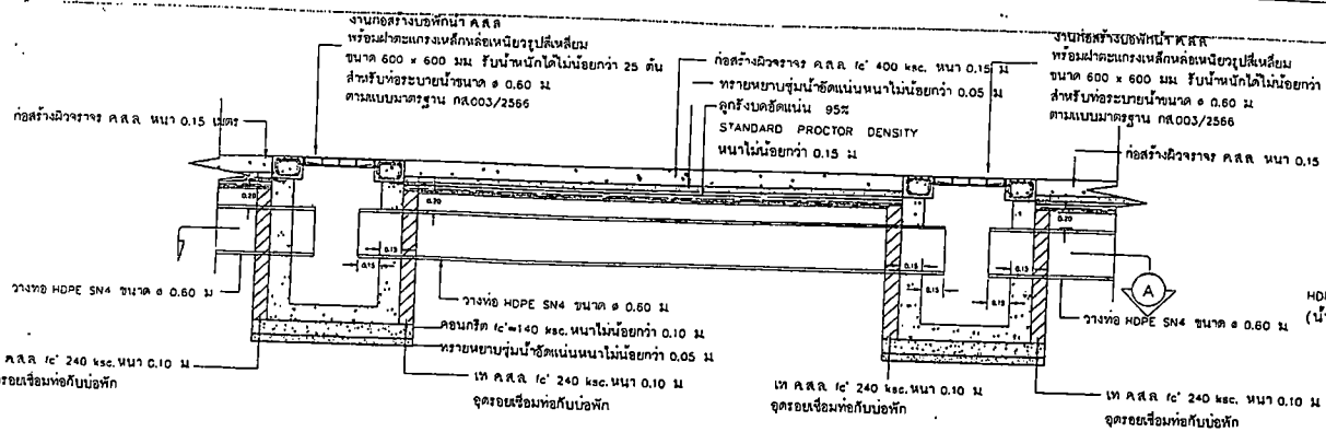
รูปตัด 4 NOT TO SCALE
