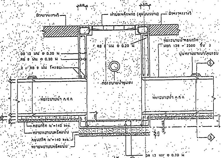
รูปตัด ① มาตราส่วน 1:20
