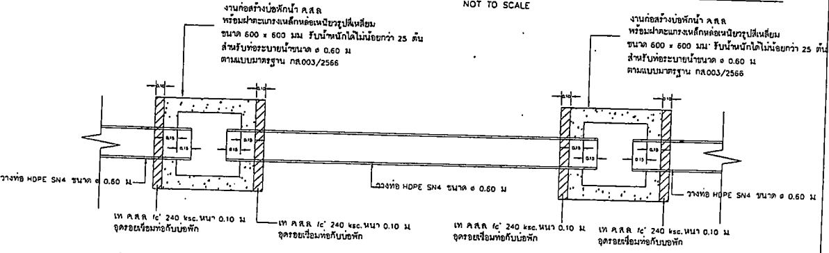
รูปตัด A NOT TO SCALE
