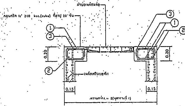
รูปตัด B - B NOT TO SCALE
