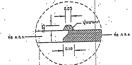
แบบขยายการแนวรอยต่อ not to scale
