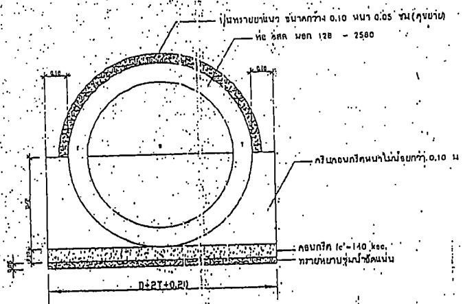
รูปตัด ๕ มาตรฐาน 1 : 10
