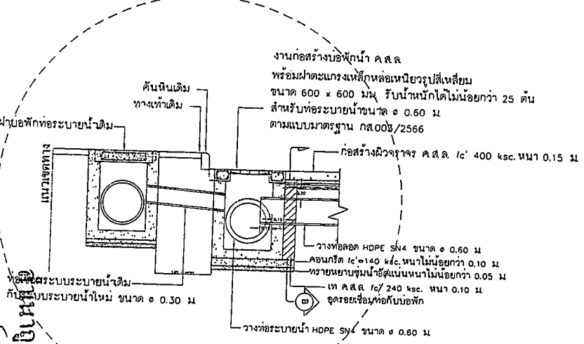
รูปตัด B NOT TO SCALE
