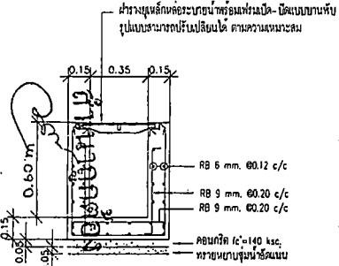
รูปตัด 1 มาตราส่วน 1/15
