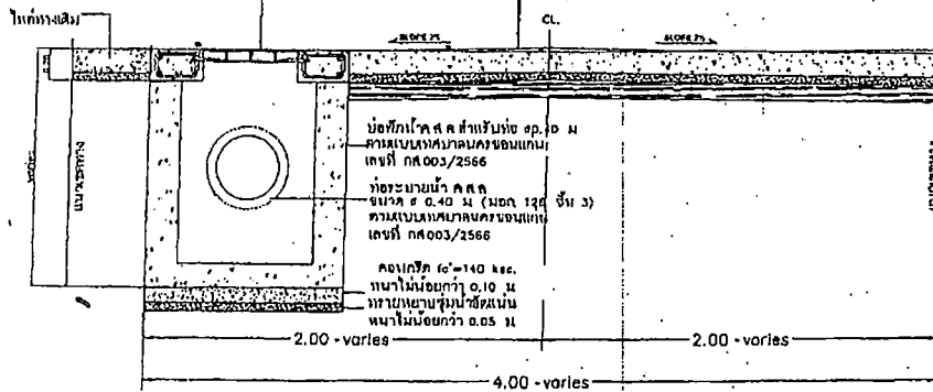
รูปตัด 1 NOT TO SCALE
