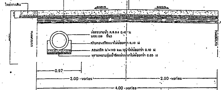
รูปตัด 2 NOT TO SCALE
