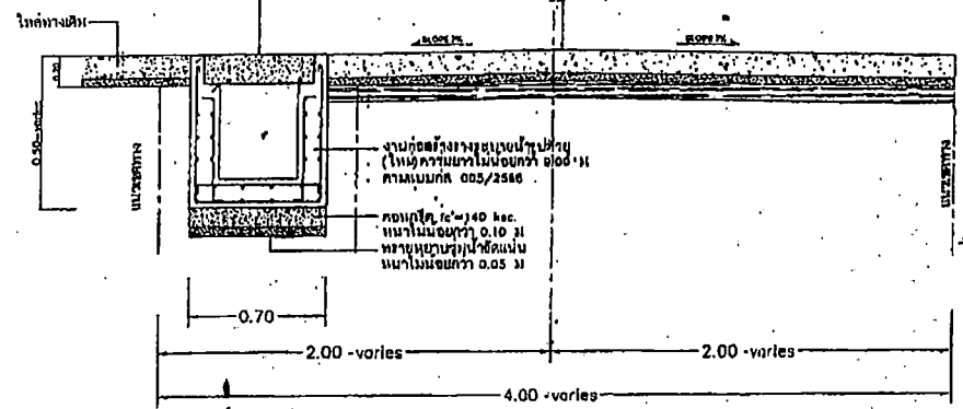
รูปตัด 3 NOT TO SCALE
