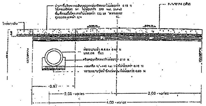
รูปตัด 2 NOT TO SCALE
