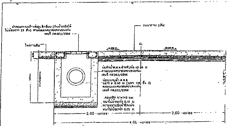
รูปตัด 1 NOT TO SCALE
