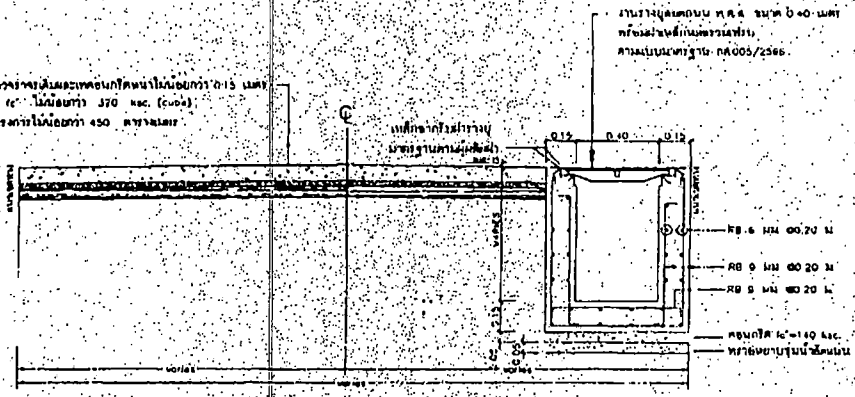
รูปตัด 1 NOT TO SCALE
