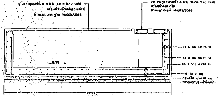
รูปตัด 3 NOT TO SCALE
