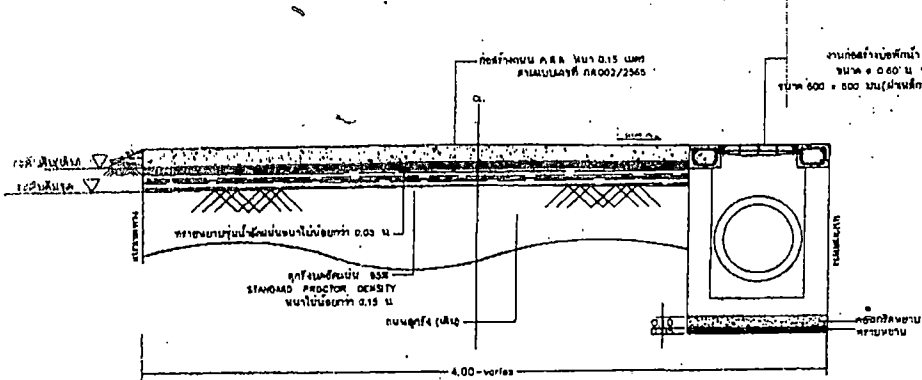
รูปตัด 2 sta. 0+075 ถึง sta. 0+115 NOT TO SCALE
