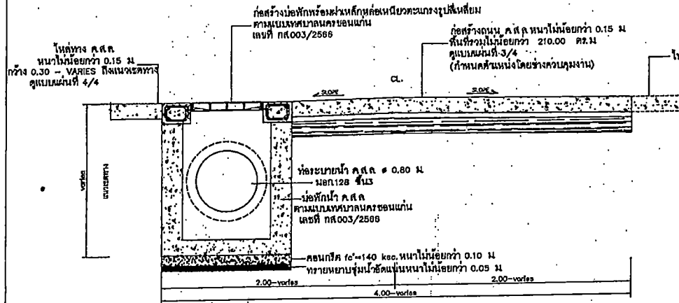
รูปตัด 1 NOT TO SCALE
