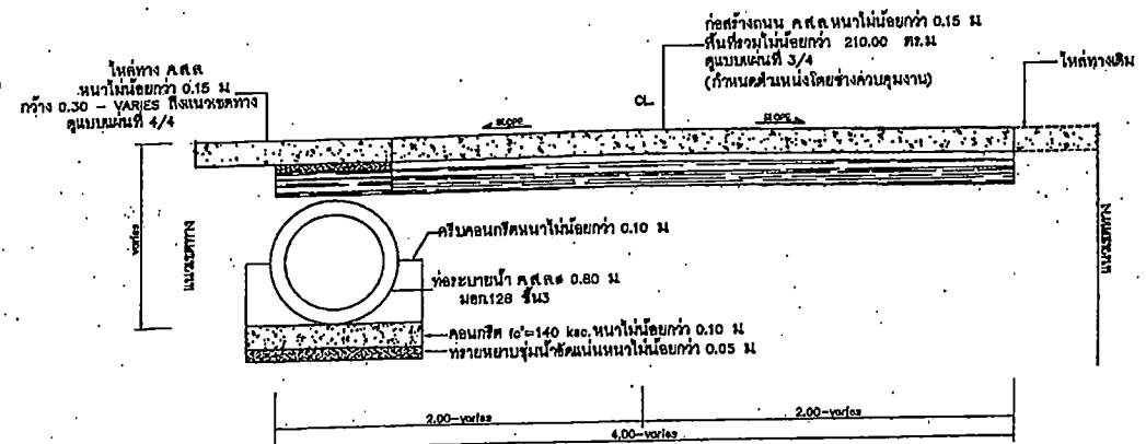
รูปตัด 2 NOT TO SCALE
