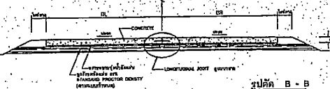
รูปตัด B-B NOT TO SCALE
