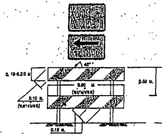
แผงกั้น 2 แฉก สำหรับเบี่ยงซ้าย ไม่แสดงขนาดฐาน
