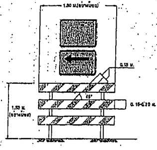
แผงกั้น 3 แฉก สำหรับเบี่ยงซ้าย ไม่แสดงขนาดฐาน
