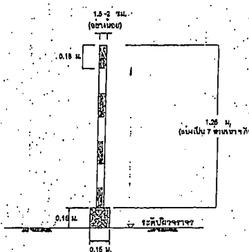
หลักกิโลเมตร ไม่แสดงขนาดฐาน
