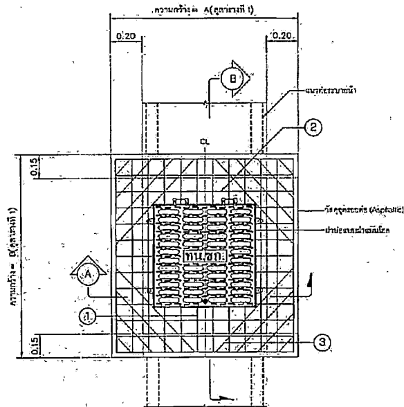
แปลนเหล็กเสริมโครงสร้างยึดพาดูพื้หน้าเหล็กหล่อเหนียว NOT TO SCALE
