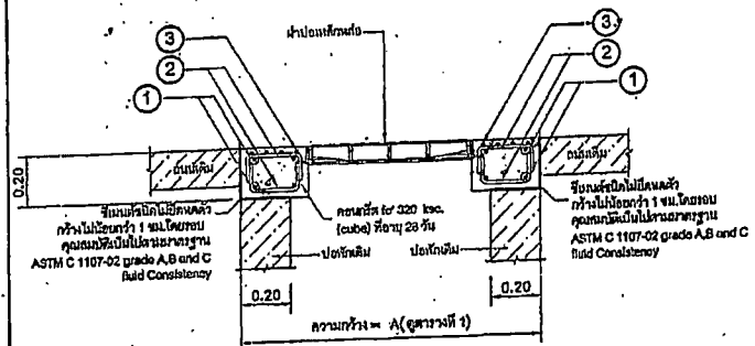
รูปตัด A-A NOT TO SCALE
