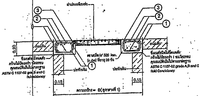
รูป.ตัด B-B NOT TO SCALE
