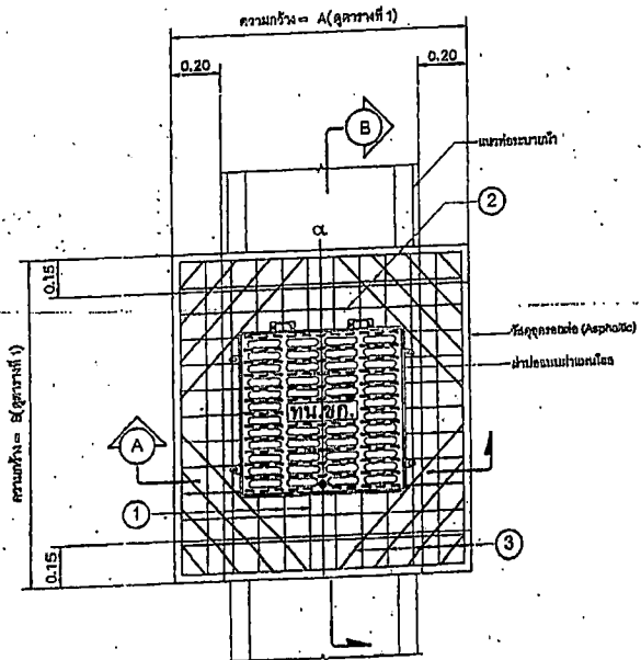
แปลนเหล็กเสริมโครงสร้างยึดฝาป่อเหล็กหล่อเหนียว
