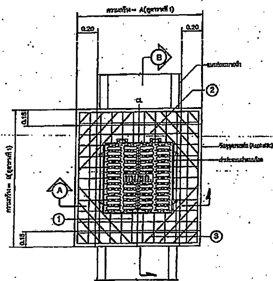
แปลนเหล็กเสริมโครงสร้างปิดฝาลอเหล็กหล่อเหนียว NOT TO SCALE
