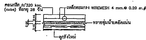
ขยายให้สัทาง ค.ส.ล. หน้าไม่น้อยกว่า 0.15 ม. NOT TO SCALE
