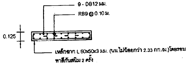
รูปตัดฝ่าบ่อพัก ไม่ได้มาตรฐาน
