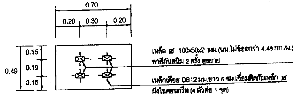
แปลนฝ่าบ่อพัก ไม่ได้มาตรฐาน
